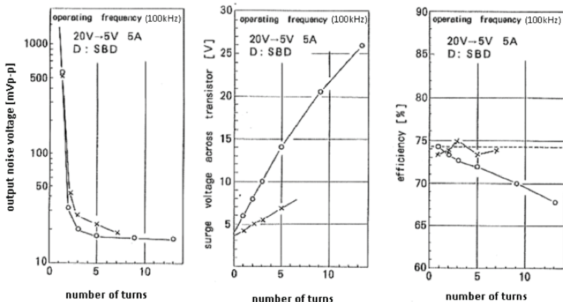
7-1) Output noise
